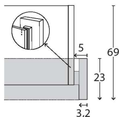
Draufsicht Schrank inkl. PPT-Rahmen
